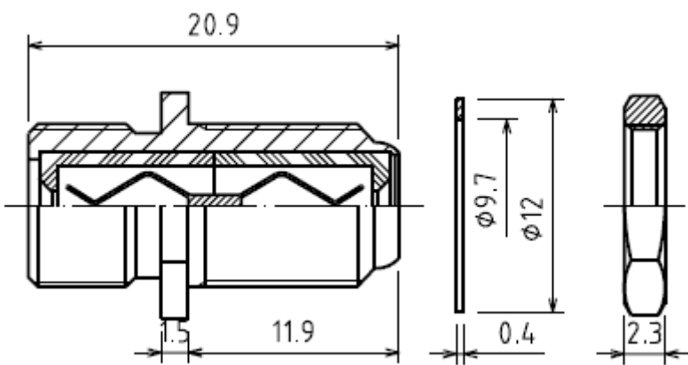
Схема изделия
