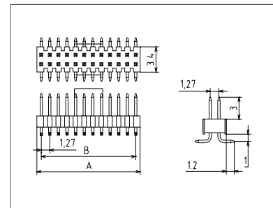
PLLD1.27-xxS xx—количество контактов
