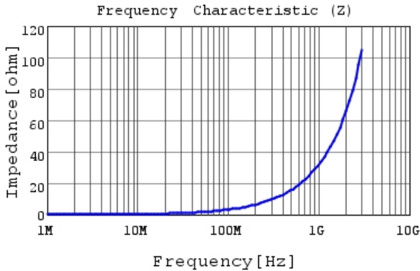
LQW15AN5N1G8Z |Z|
