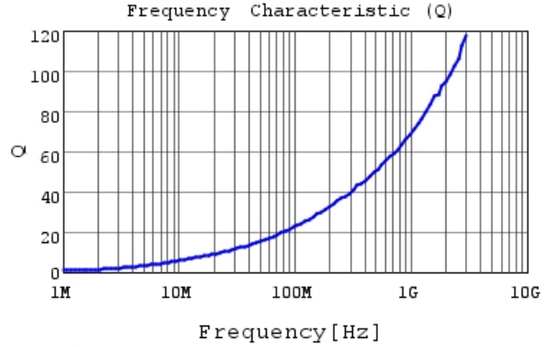
LQW15AN3N6G8Z Q
