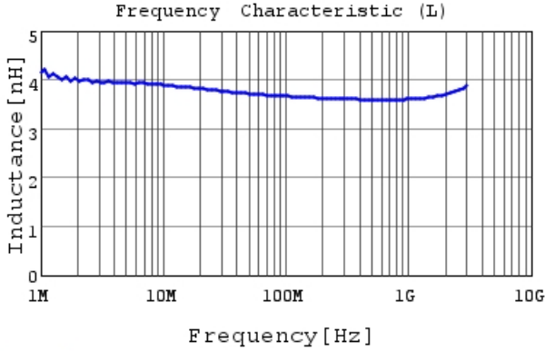
LQW15AN3N6G8Z L
