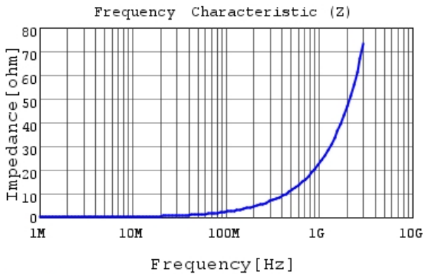
LQW15AN3N6G8Z |Z|
