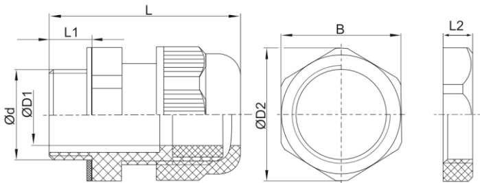
Рисунок 1. Основные размеры сальников
