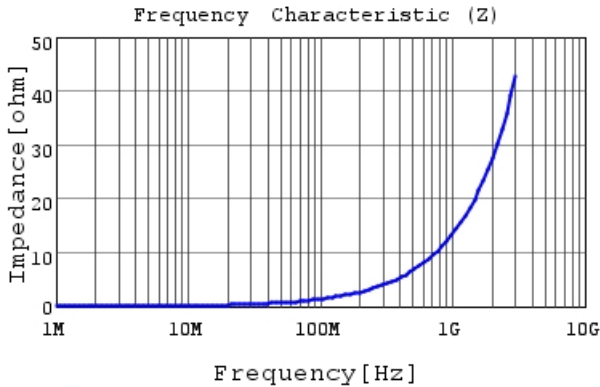
LQW15AN2N2G8Z |Z|
