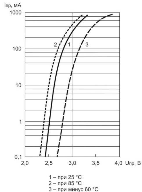
Прямая ветвь ВАХ для индикаторов КИПД162А9-С
