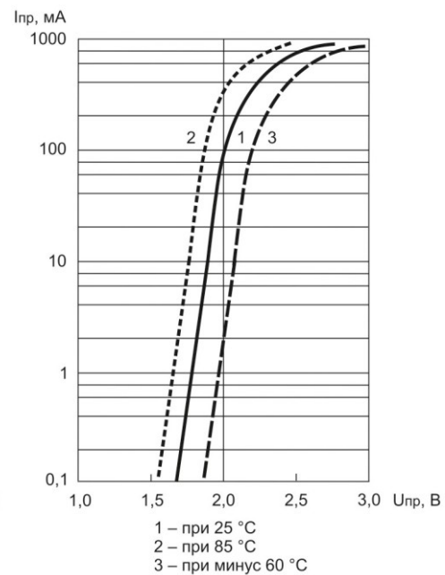
Прямая ветвь ВАХ для индикаторов КИПД162А9-Ж
