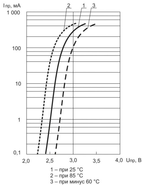
Прямая ветвь ВАХ для индикаторов КИПД160А9-С
