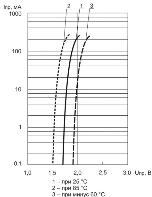
Прямая ветвь ВАХ для индикаторов ИПД160А9-Ж
