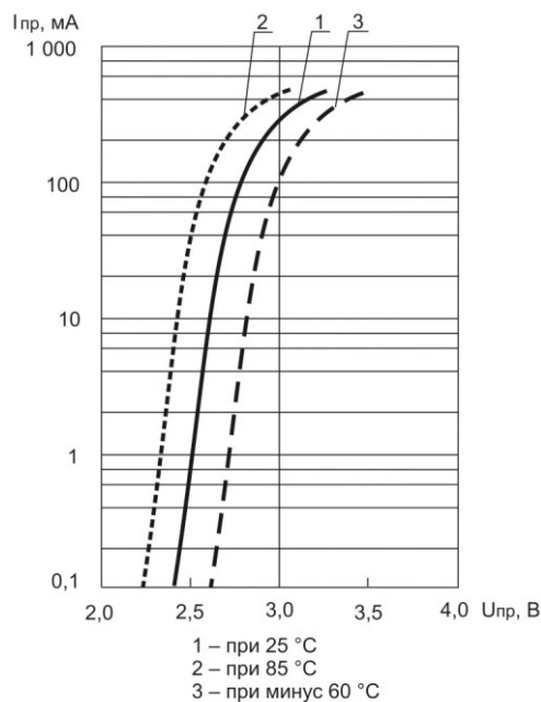
Прямая ветвь ВАХ для индикаторов ИПД160А9-С
