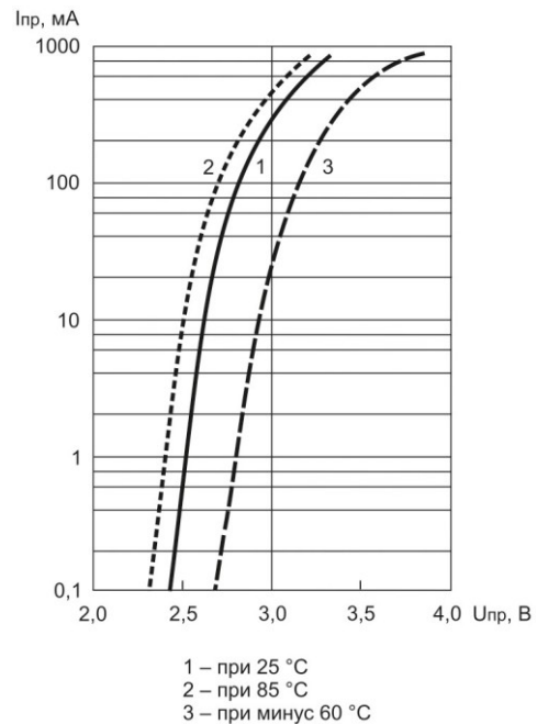
Прямая ветвь ВАХ для индикаторов ИПД162А9-С
