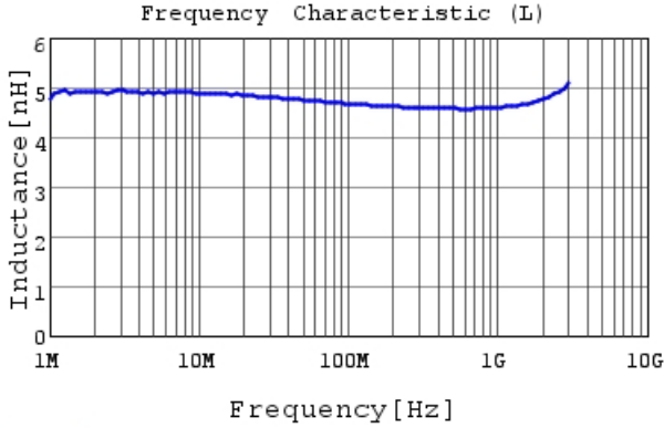
LQW15AN4N7G8Z L
