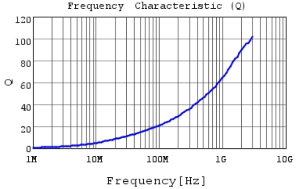
LQW15AN4N7G8Z Q
