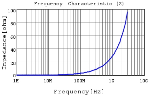
LQW15AN4N7G8Z |Z|
