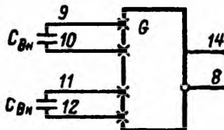
Условное графическое обозначение К218ГГ1
