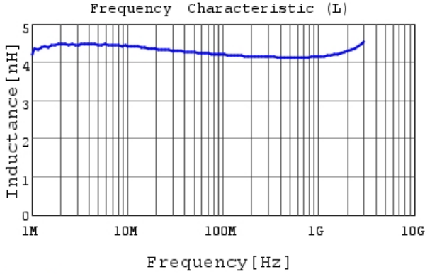
LQW15AN4N3G8Z L
