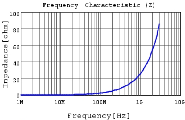
LQW15AN4N3G8Z |Z|
