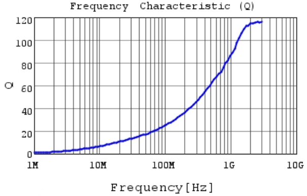
LQW15AN4N3G8Z Q
