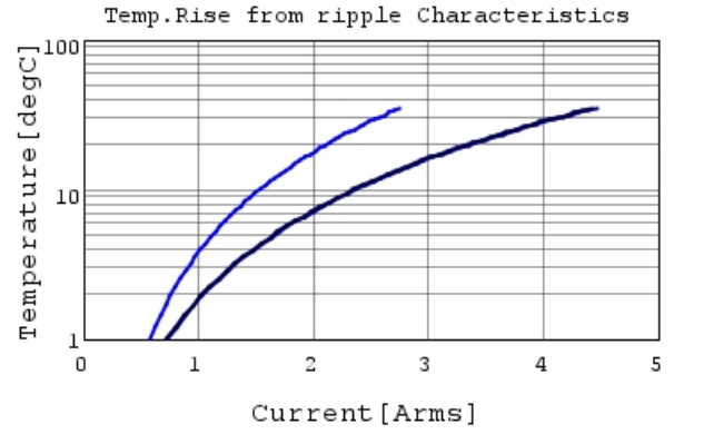
GRM31MR71E225KA93 Temp.rise — 100kHz —
