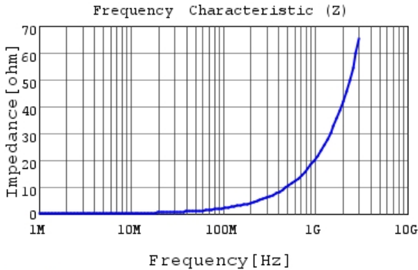
LQW15AN3N3G8Z |Z|
