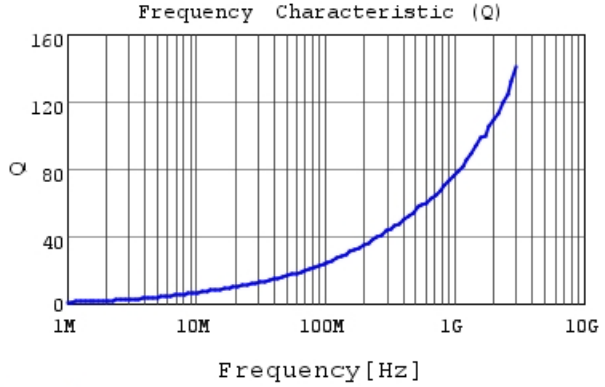
LQW15AN3N3G8Z Q
