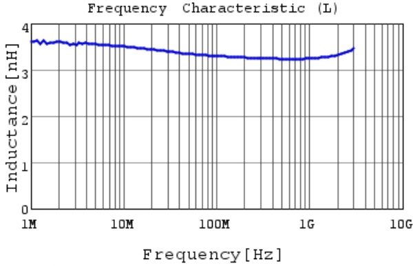
LQW15AN3N3G8Z L
