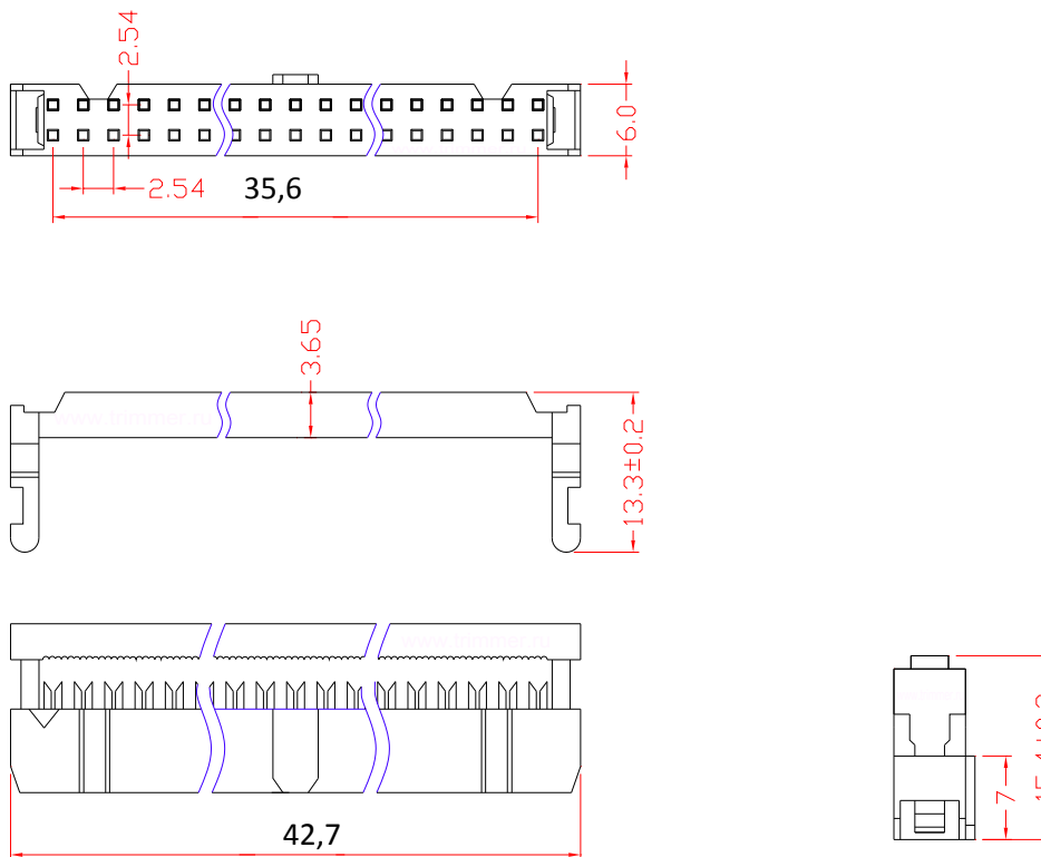
ЧЕРТЕЖ разъема IDC-30F розетка
