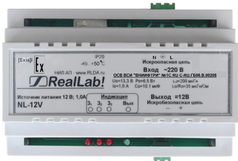
Рис. 1.2. Источник питания NL-12V, взрывозащищённого исполнения. Вид сверху.
