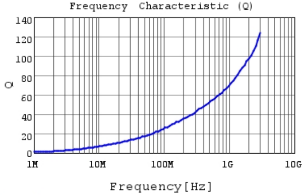
LQW15AN2N4G8Z Q
