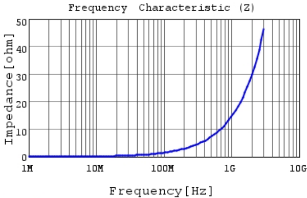
LQW15AN2N4G8Z |Z|
