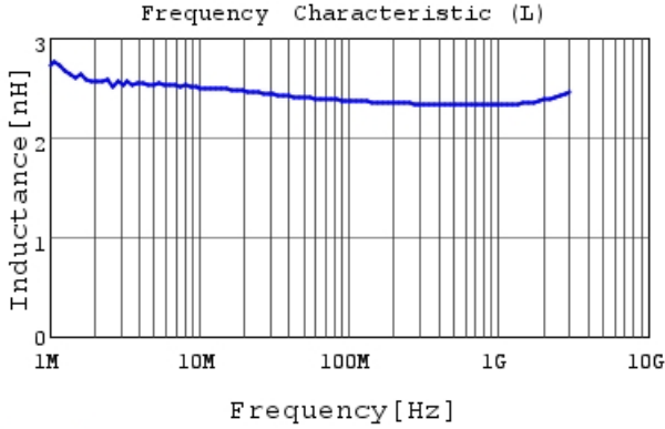
LQW15AN2N4G8Z L
