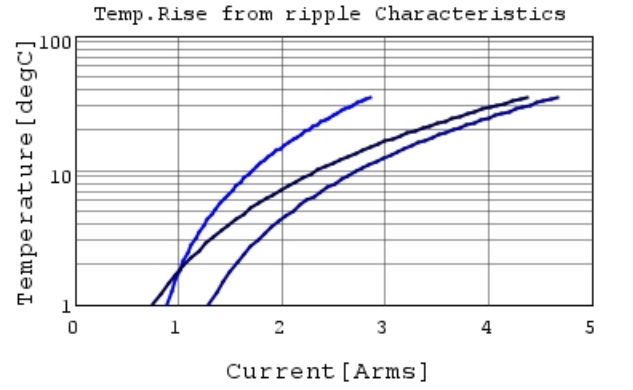
GRM31CR71H225KA88 Temp.rise 100kHz
